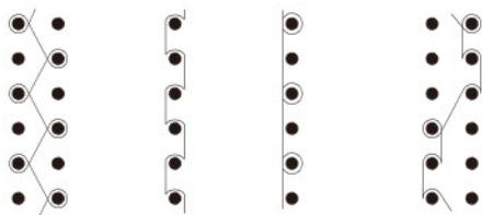
經編織圖 Warp Transmitting Pattern
